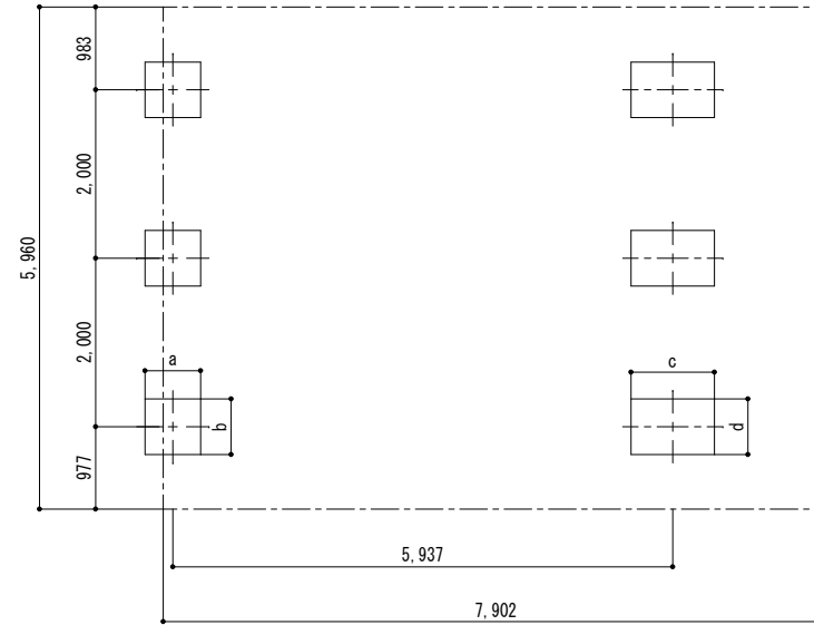
■ 基礎配置図
